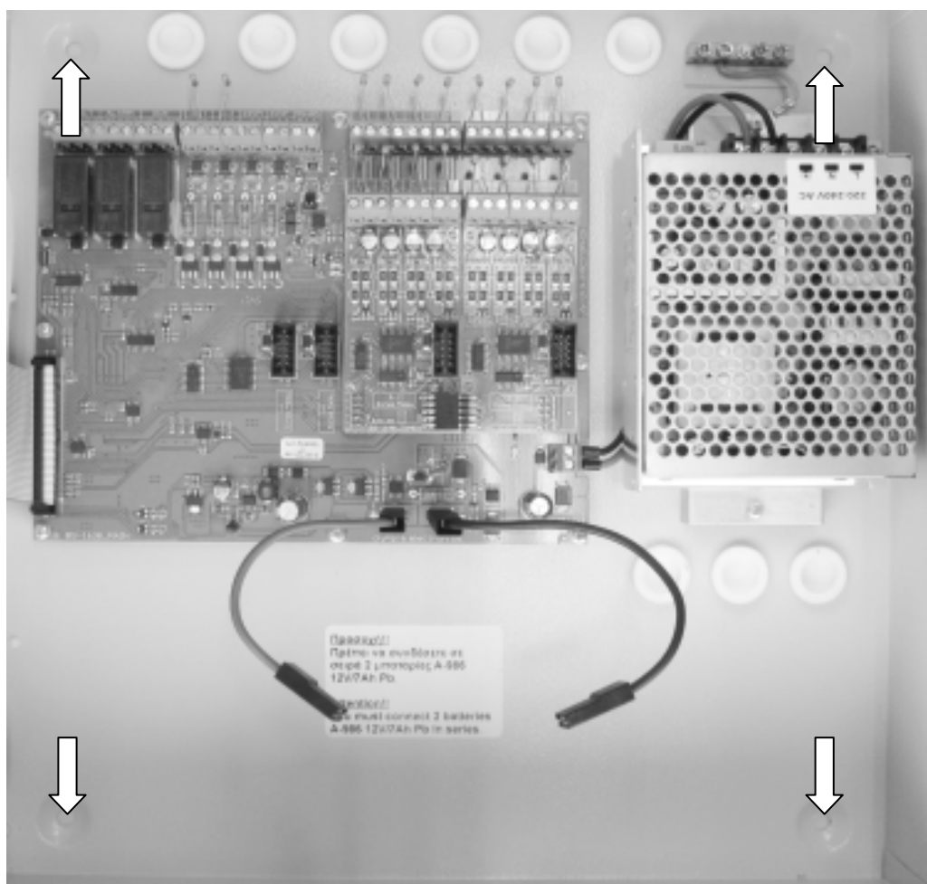
Εικόνα 4-1. Πίσω όψη του πίνακα.
