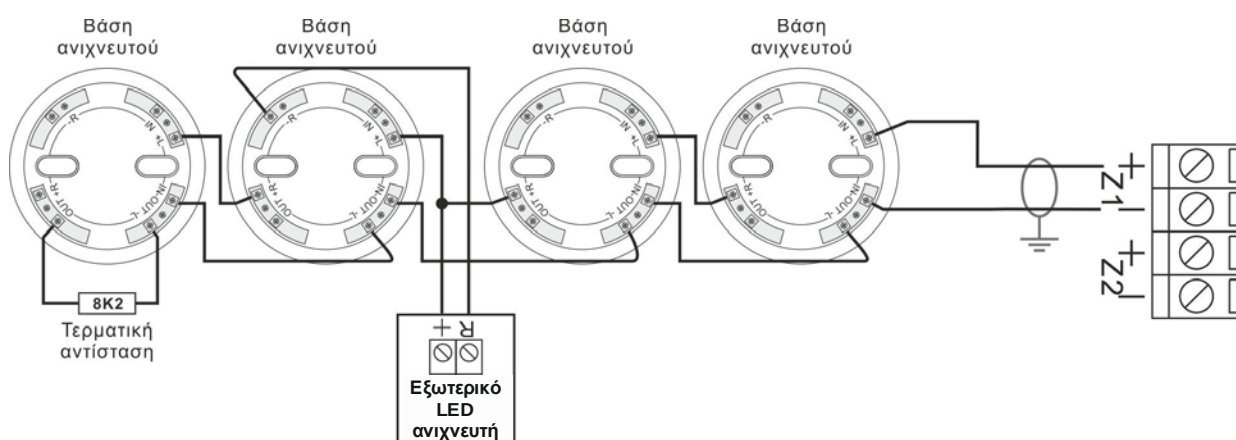
Σχ. 4-5. Σύνδεση 4 βάσεων ανιχνευτών στη ζώνη 1. Στην κάθε βάση μπορεί να τοποθετηθεί ανιχνευτής BS-655/MAR, BS-660/MAR ή BS-657/MAR. Σε έναν ανιχνευτή είναι συνδεδεμένο ένα εξωτερικό LED ανιχνευτή.
