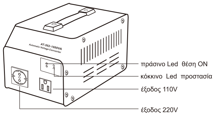
AT-502-500VA~1000VA
