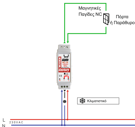
ΣΥΝΔΕΣΜΟΛΟΓΙΑ AC-16
