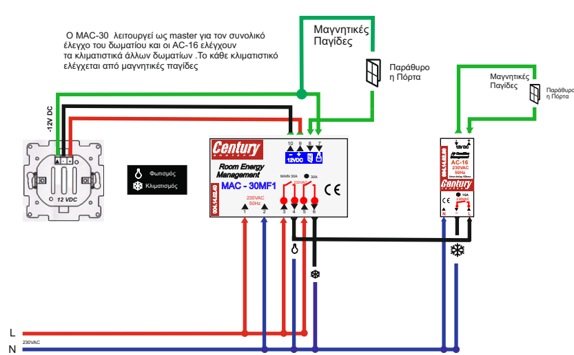
ΣΥΝΔΕΣΜΟΛΟΓΙΑ MAC-30MF1 ΣΕ ΣΥΝΔΙΑΣΜΟ ΜΕ AC-16 RFID 13,56 MHz
