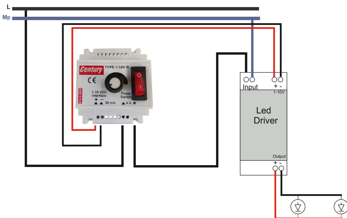
Συνδεσμολογία controller 1-10V
